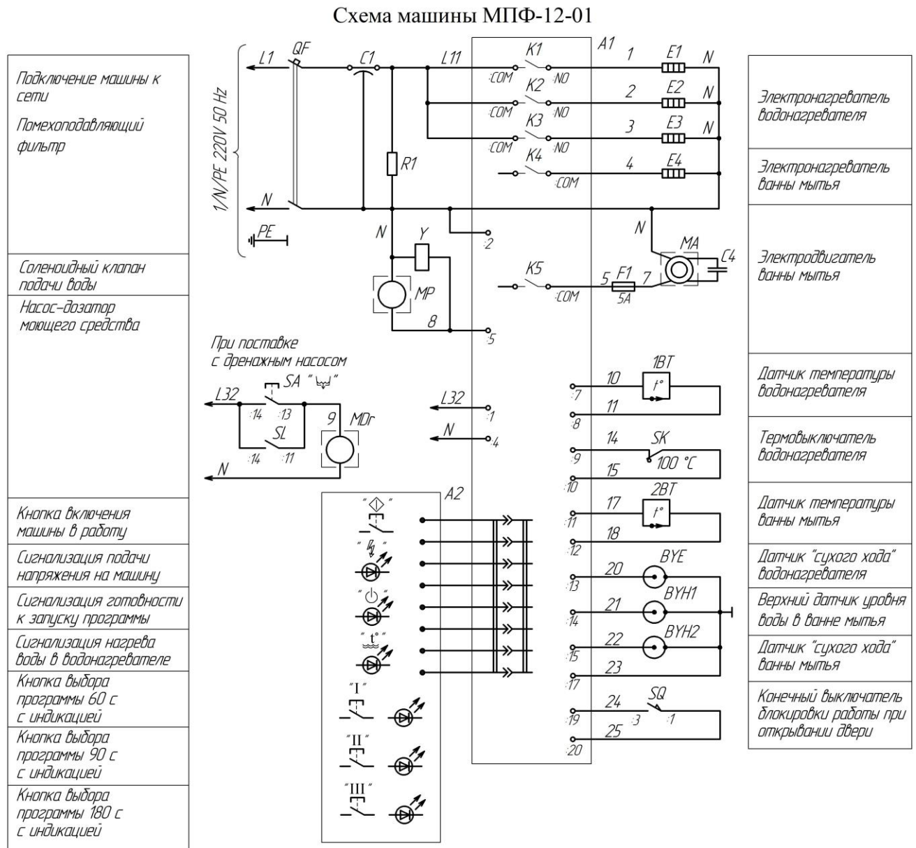
Схема машины МПФ-12-01-3 Остальное - см. схему МПФ-12-01
