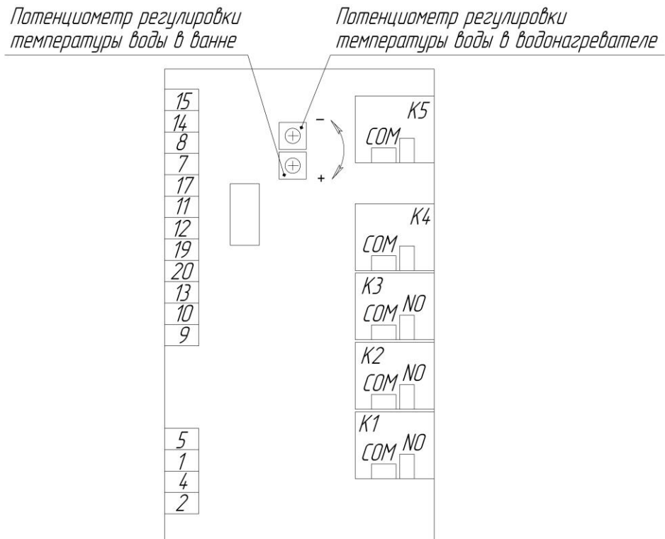
Рисунок 2 – Условное обозначение контактов блока управления
